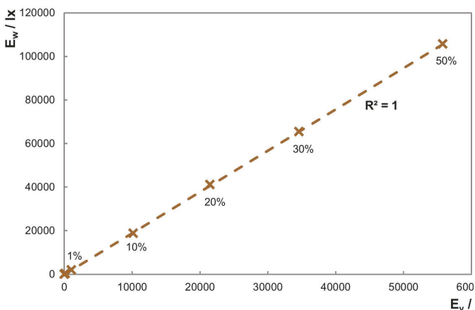
Abbildung 2: Lineare Abhängigkeit des Signals E_W des Actiwatch Spectrum-Detektors SN 08992 von der Beleuchtungsstärke E_V . In der Abbildung wurde auch die Transmission der angewendeten Neutraldichtefilter angegeben.
