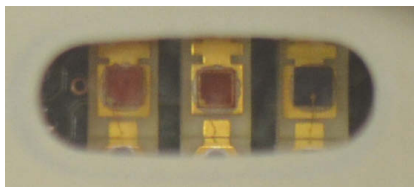
Abbildung 3a: Positionierung der R-, G- und B-Sensoren im Gehäuse der Actiwatch Spectrum-Detektoren.
