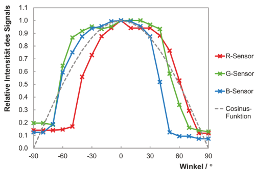
Abbildung 3b: Gemessene horizontale Richtungsempfindlichkeit der R-, G- und B-Sensoren des Actiwatch Spectrum-Detektors SN 08968 im Vergleich zur Cosinus-Funktion.
